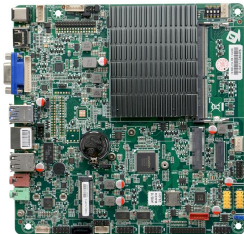
ITX-B420_J112L VER:1.0 主板正面图
